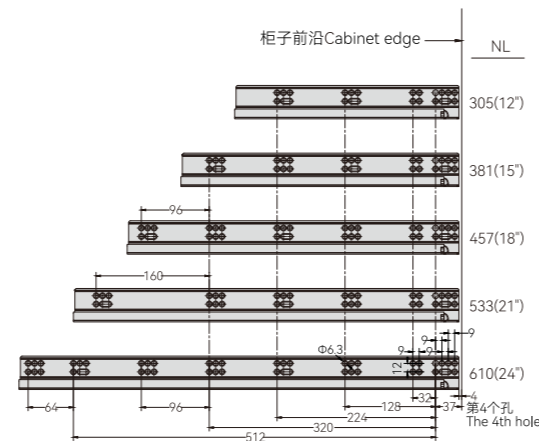
滑轨安装孔的位置(mm) Hole position
