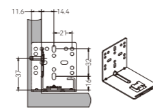
A(金属连接件)(Metal bracket)
