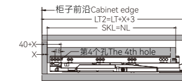
内置抽屉 Internal drawer
