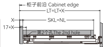
内置抽屉 Internal drawer
