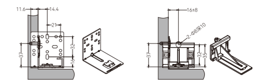
A(金属连接件)(Metal bracket)
