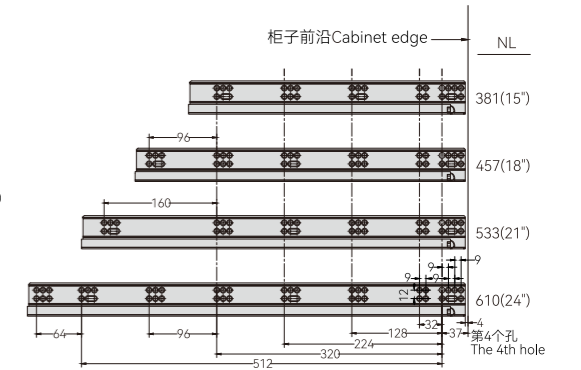
滑轨安装孔的位置(mm) Hole position
